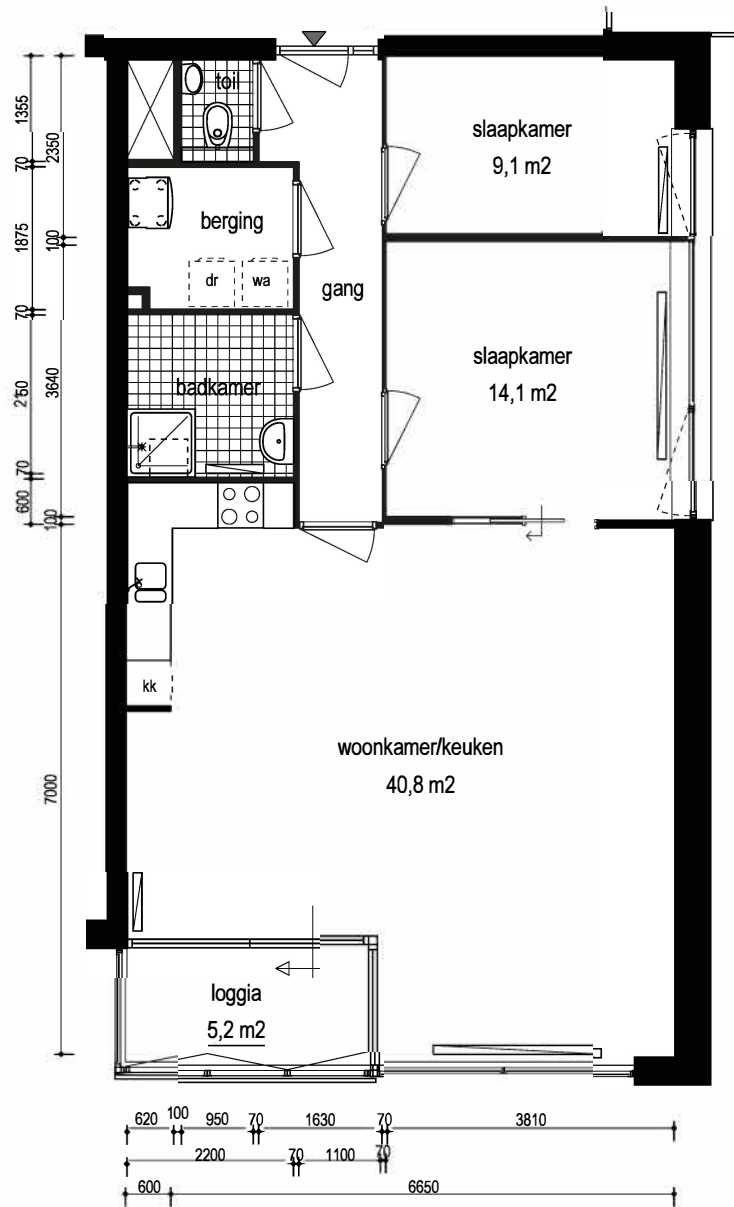
woningtype A'
